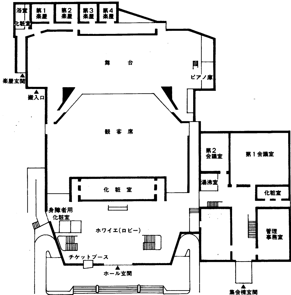
1階平面図
